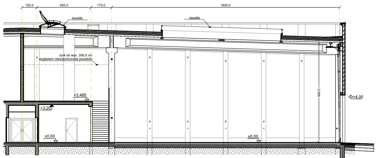
Poglądowy przekrój
