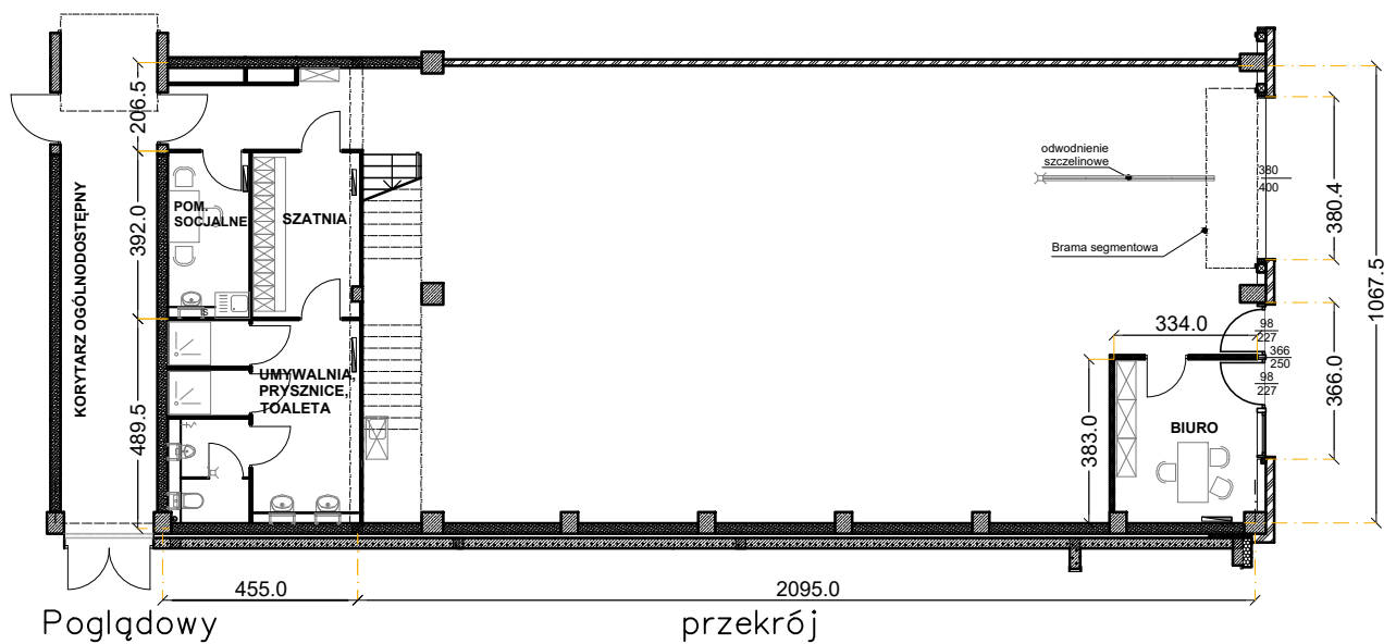
Rzut parteru
