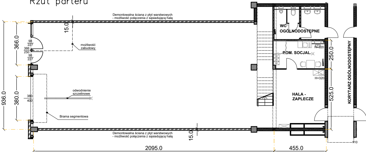
Rzut parteru
