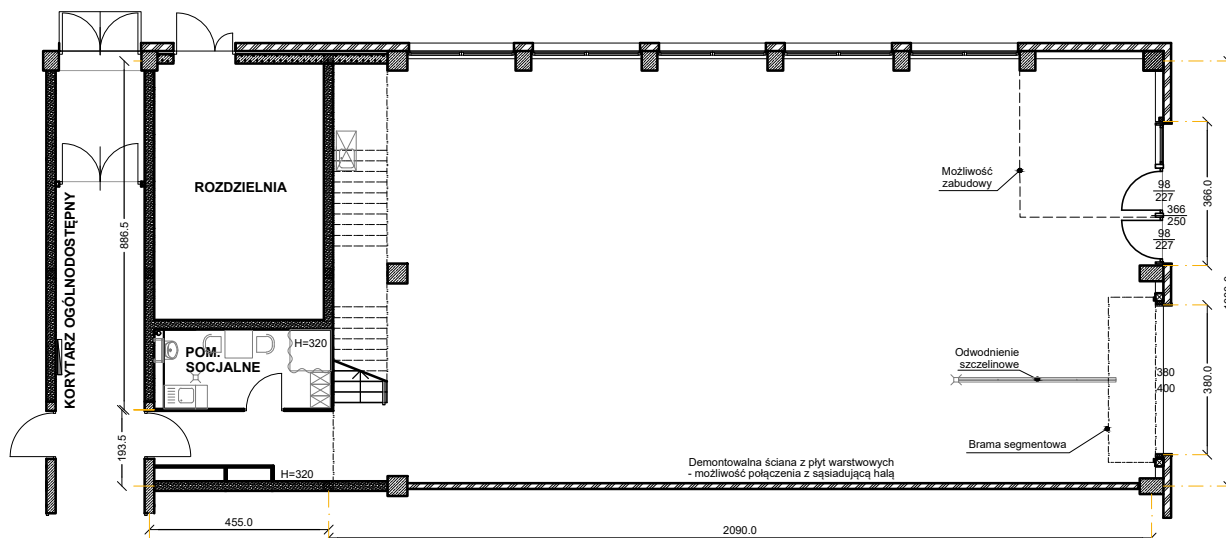
Rzut parteru
