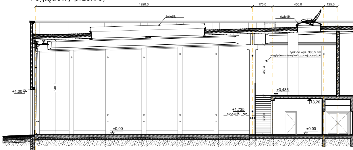
Poglądowy przekrój
