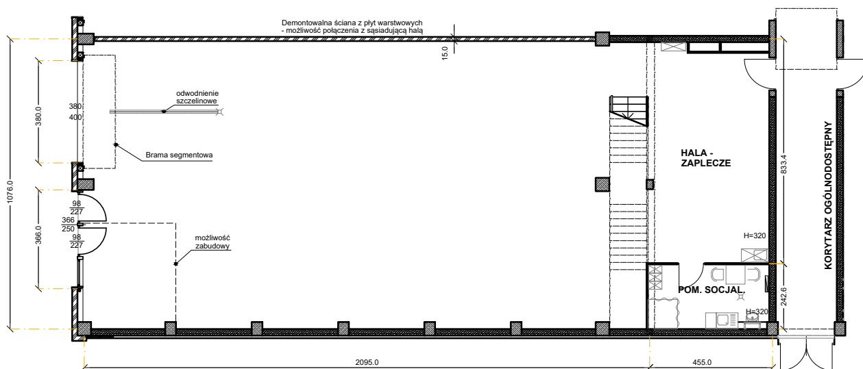
Rzut parteru
