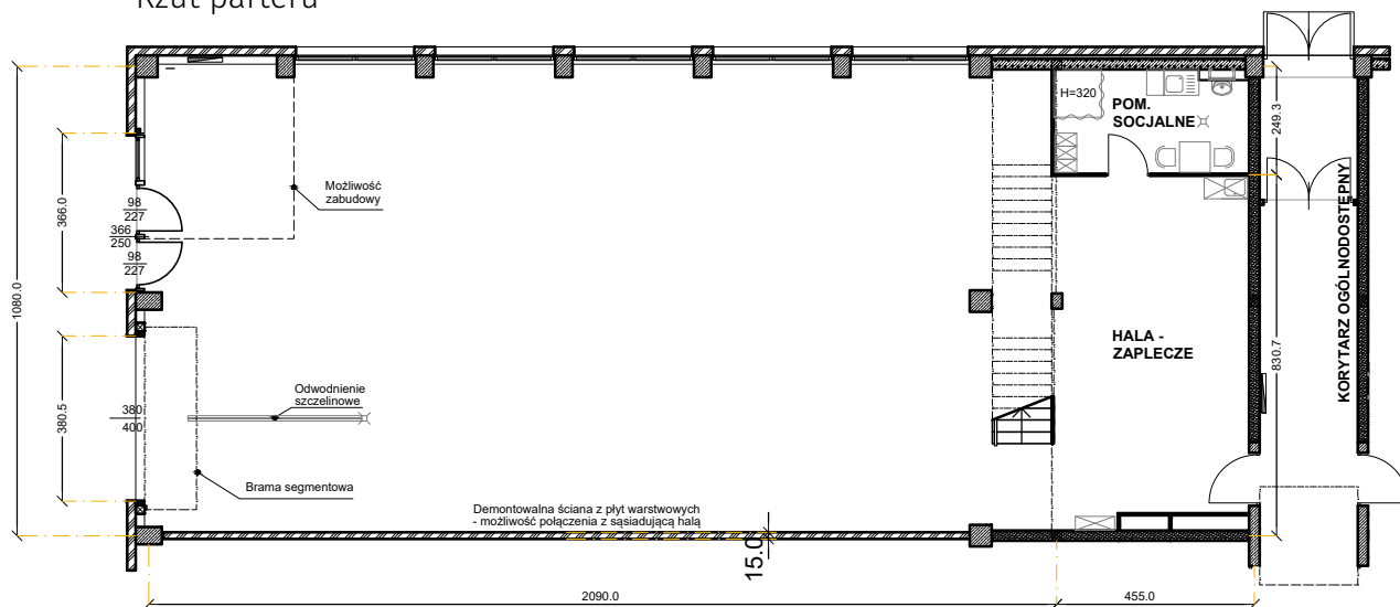
Rzut parteru
