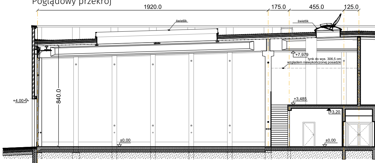
Poglądowy przekrój
