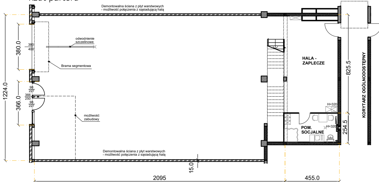
Rzut parteru
