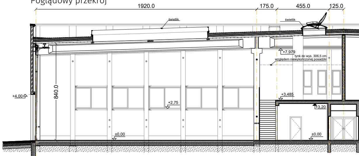
Poglądowy przekrój
