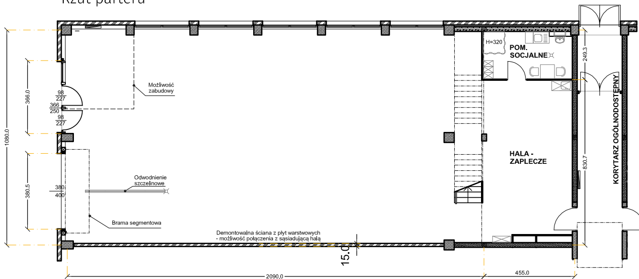
Rzut parteru
