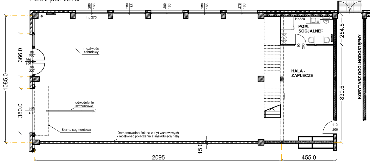
Rzut parteru
