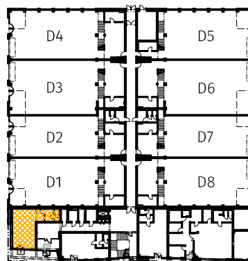
Rzut sytuacyjny
