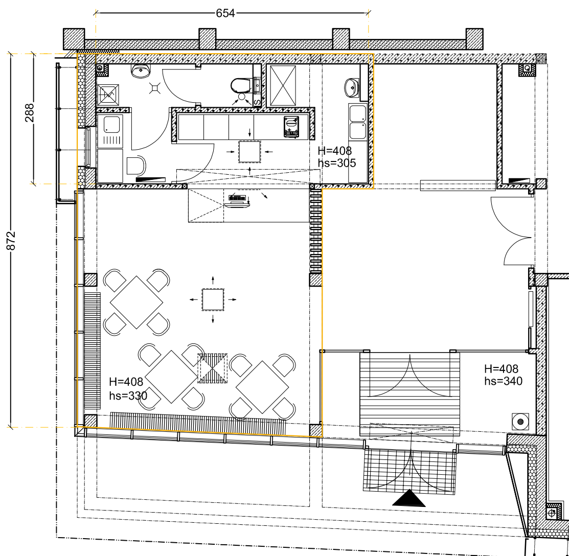
Poglądowy rzut bistro
